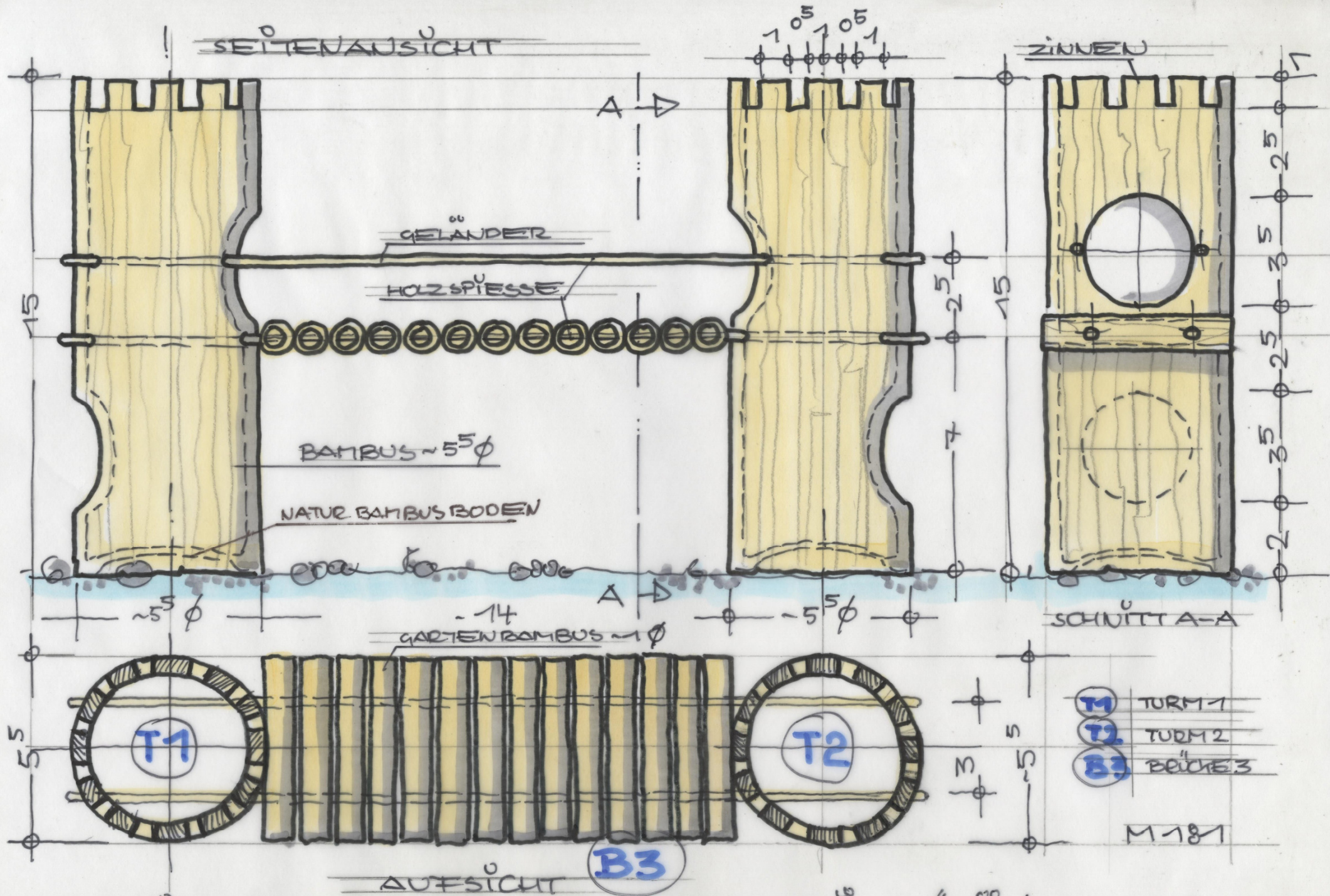
ANSICHTEN UND SCHNITT "BAMBUS BRÜCKE" FÜR'S AQUARIUM
